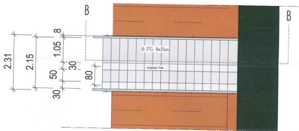
DRAUFSICHT KINDERWAGENTREPPE
